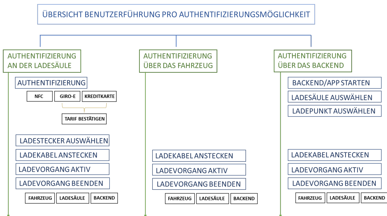
Abbildung 54: Übersicht Benutzerführung pro Authentifizierungsmöglichkeit
