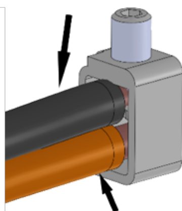
Abbildung 30: Anbringung Kabelklemmen
