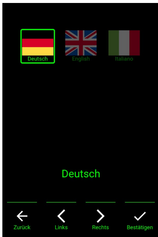
Abbildung 57: Sprachauswahl
