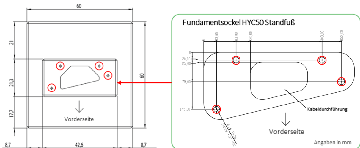
Abbildung 19: Positionierung Standfuß auf Fundament
